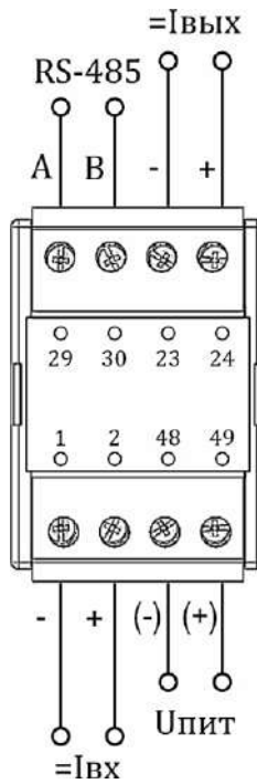
в) Корпус M8 (1 вход, 1 аналоговый выход, 1 порт RS-485)
